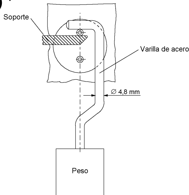
Figura 14 – Dispositivo de ensayo de las espigas no macizas
