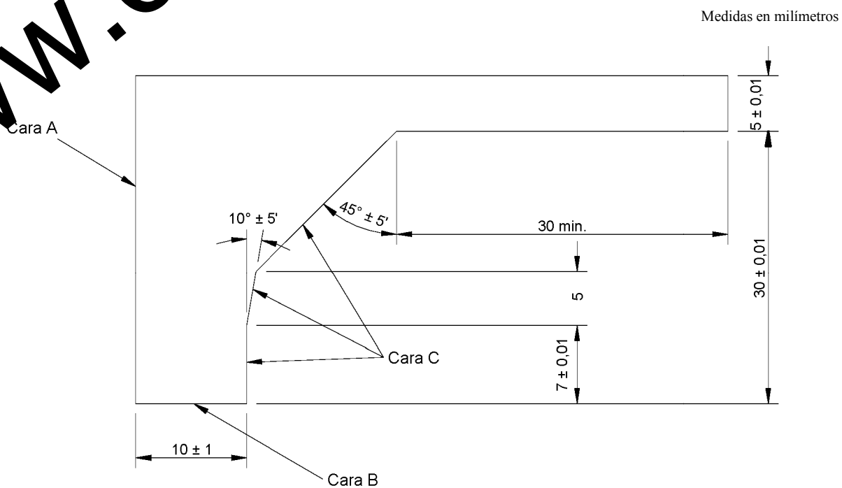
Figura 32 – Calibre (espesor: 2 mm aproximadamente) para la verificación del contorno de las tapas y placas de recubrimiento
