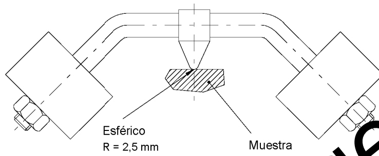
Figura 37 – Aparato para el ensayo de presión
