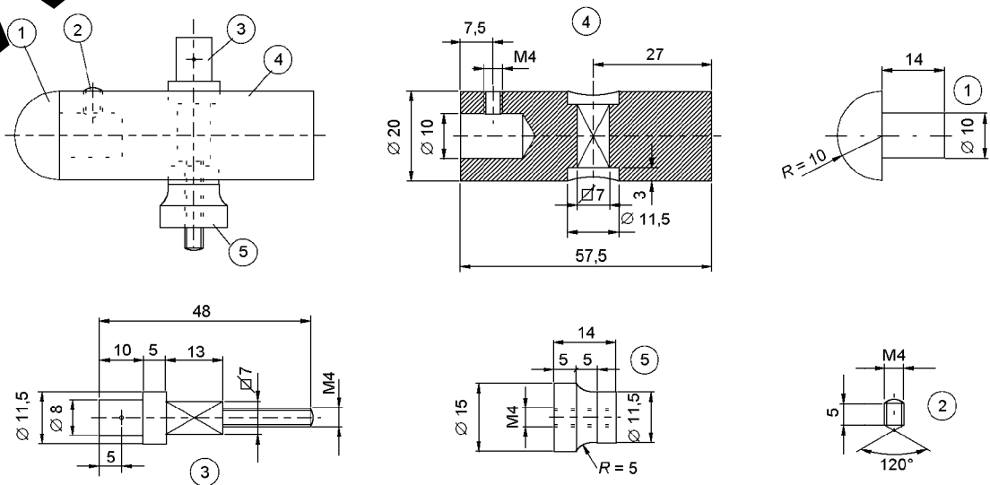
Figura 22 – Aparato para el ensayo de choque
