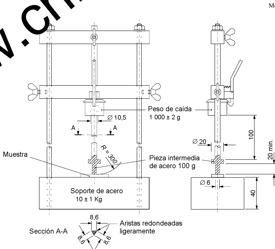
Figura 42 – Aparato de ensayo de choque sobre espigas provistas de manguitos aislantes
