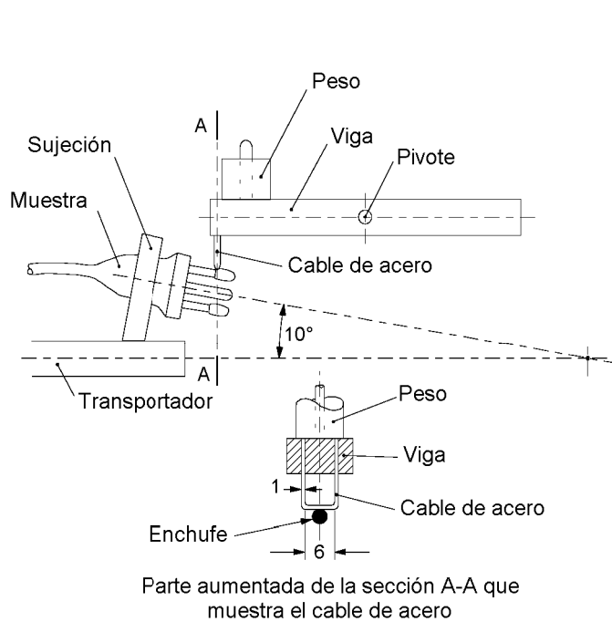
Figura 28 – Aparato para el ensayo de abrasión del manguito aislante de las espigas de las clavijas
