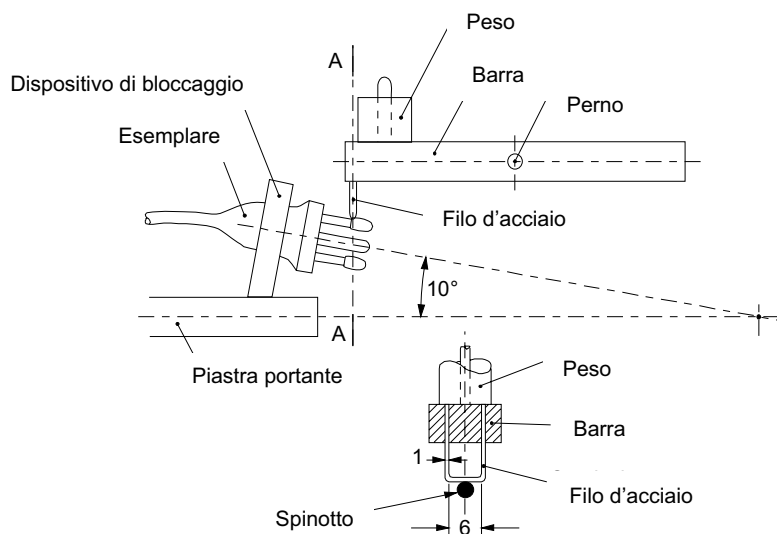
Figura 27 – Apparecchio per la prova d'urto a bassa temperatura di 24.4
